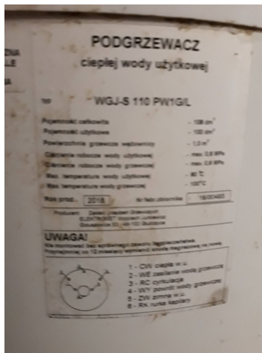
Fot. 5 . tabliczka znamionowa
