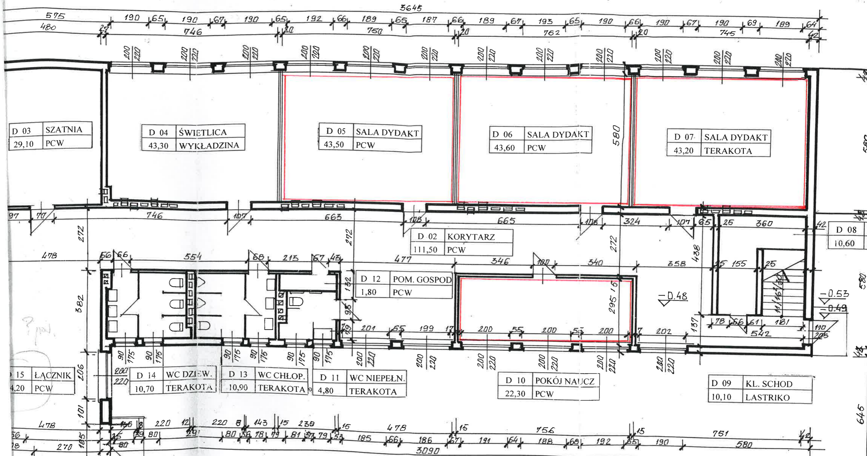
RZUT PARTERU BUDYNEK PAWILON „D” 1 : 100
