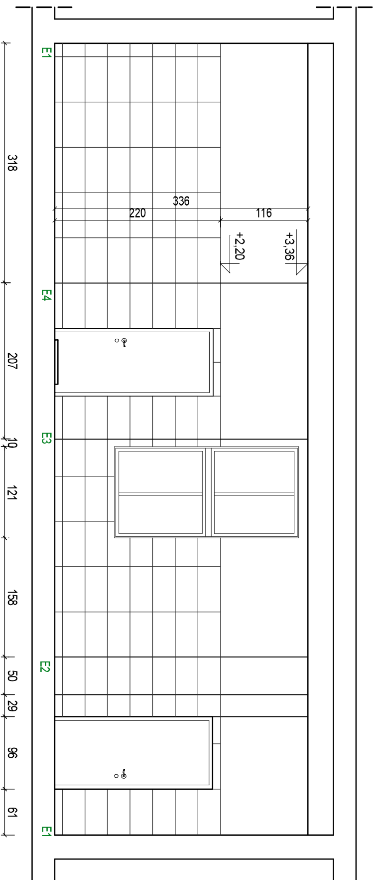
ROZWINIĘCIE ŚCIAN - PRZEDŚIONEK nr 108A 1:50
