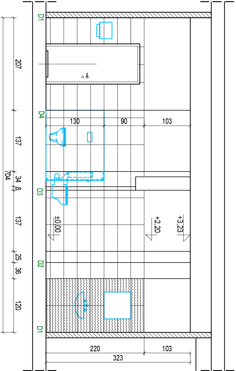
ROZWINIĘCIE ŚCIAN - TOALETA 108B 1:50
