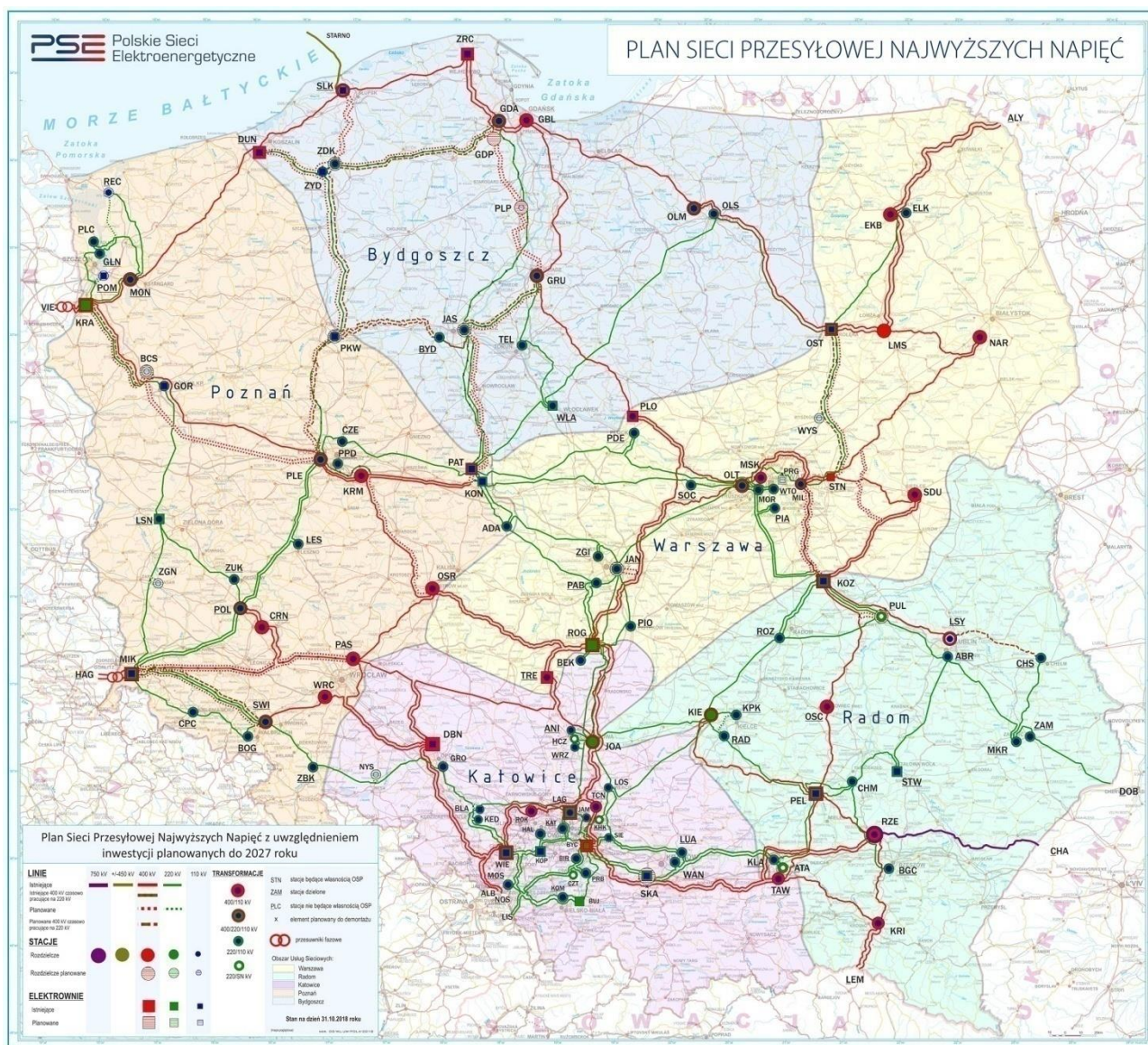
Rys. 18 Schemat Krajowego Systemu Przesyłowego (KSE)
