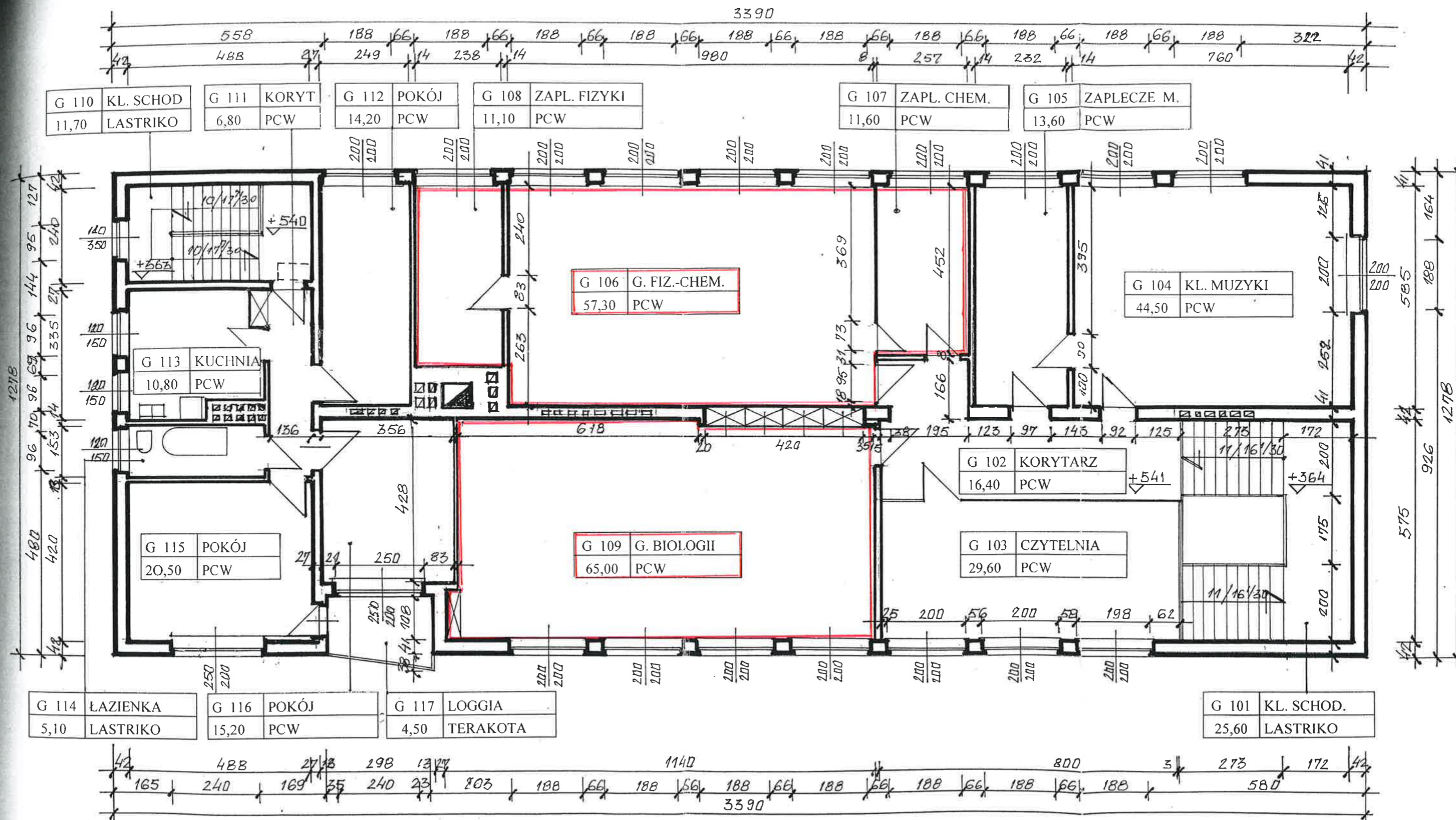
RZUT PIĘTRA BUDYNEK GŁÓWNY
