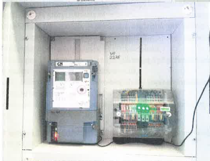
Rozdzielnica główna RG
