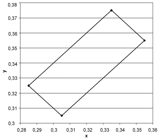
Rys. 1. Współrzędne chromatyczności x,y dla barwy białej oznakowania
