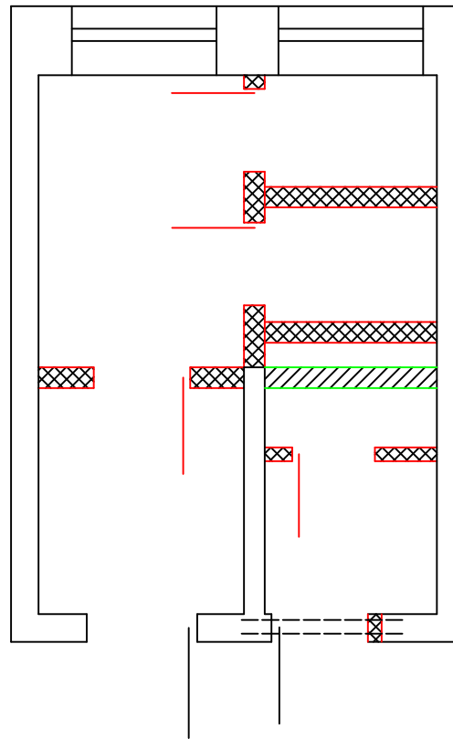
Likwidacja ścianek działowych z naświetlami i ścianek przedzielających WC
