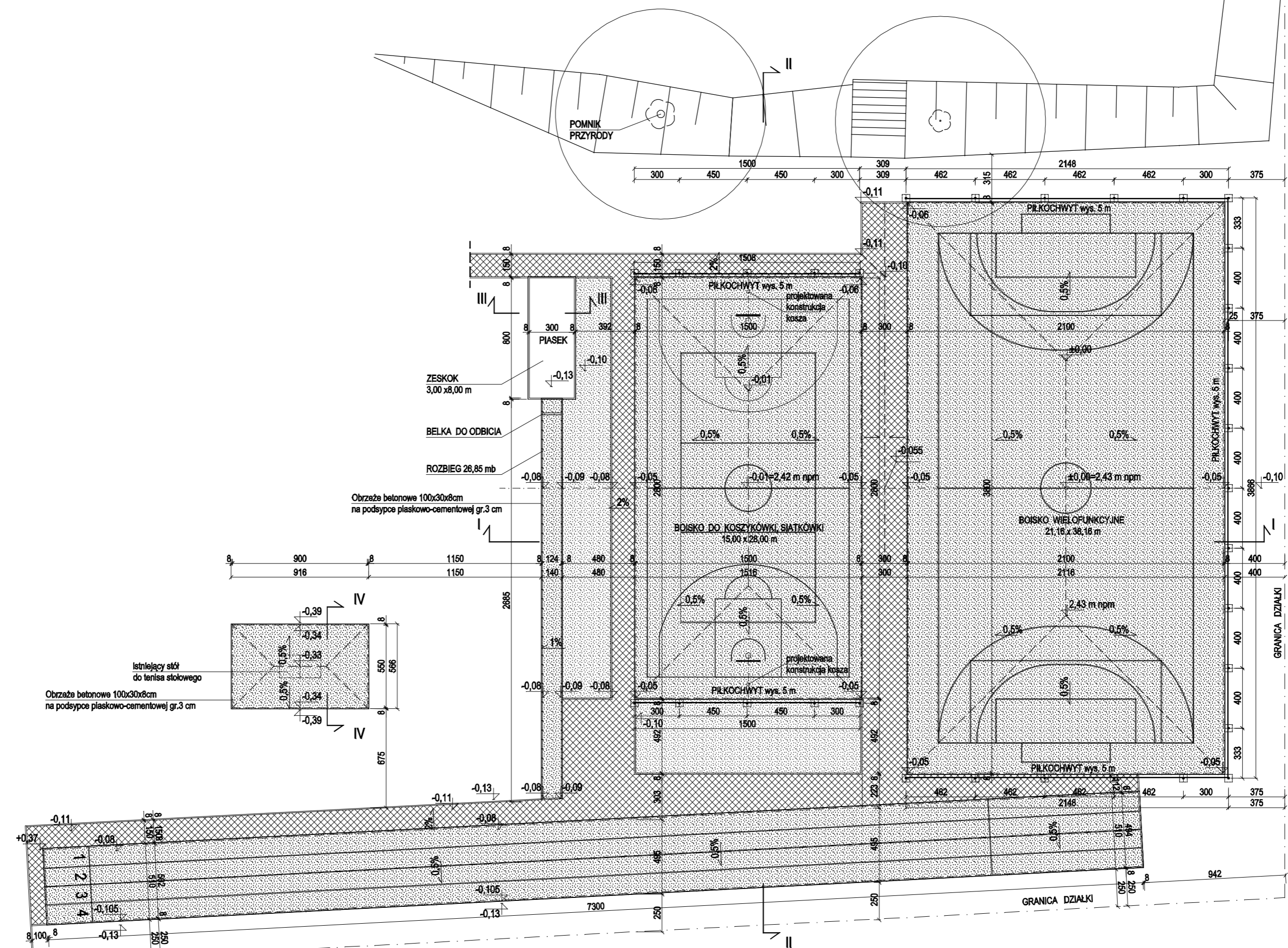
SCHEMAT LINII BOISKA, BIEŻNI 1:250
