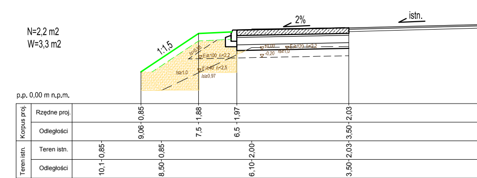
PRZEKRÓJ 2 km 0+665,80 ul. Pomorska
