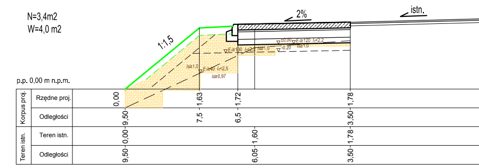
PRZEKRÓJ 3 km 0+703,40 ul. Pomorska
