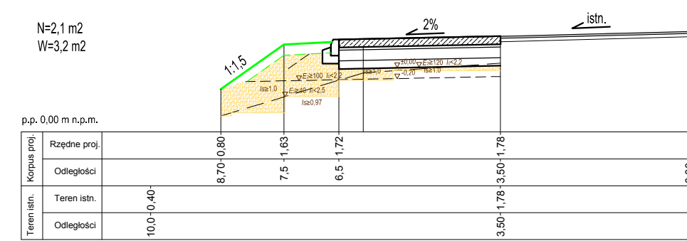
PRZEKRÓJ 4 km 0+752,50 ul. Pomorska
