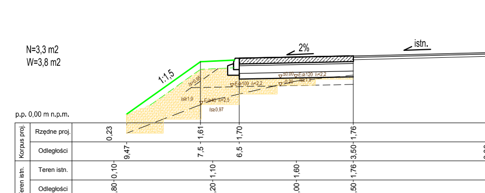
PRZEKRÓJ 6 km 0+868,20 ul. Pomorska
