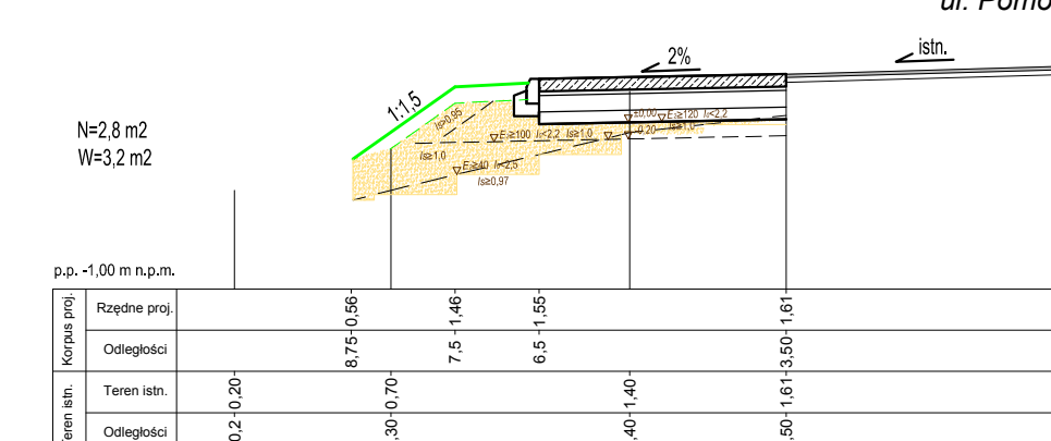
PRZEKRÓJ 14 km 1+523,80 ul. Pomorska
