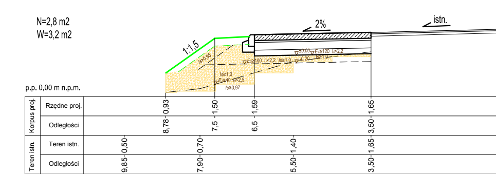
PRZEKRÓJ 13 km 1+479,85 ul. Pomorska
