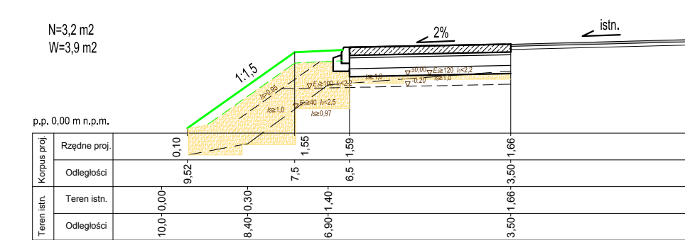
PRZEKRÓJ 7 km 0+970,90 ul. Pomorska
