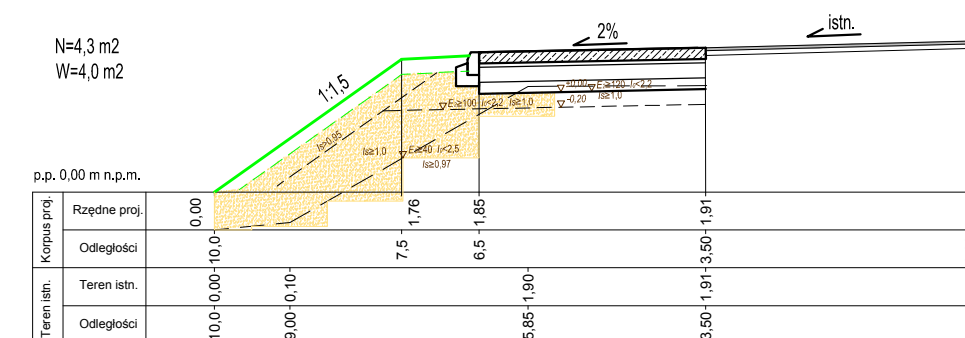
PRZEKRÓJ 2 km 0+665,80 ul. Pomorska
