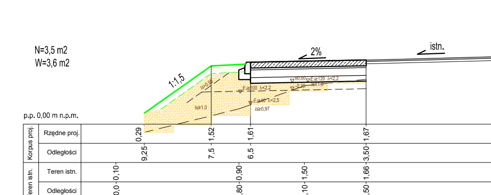
PRZEKRÓJ 9 km 1+165,75 ul. Pomorska
