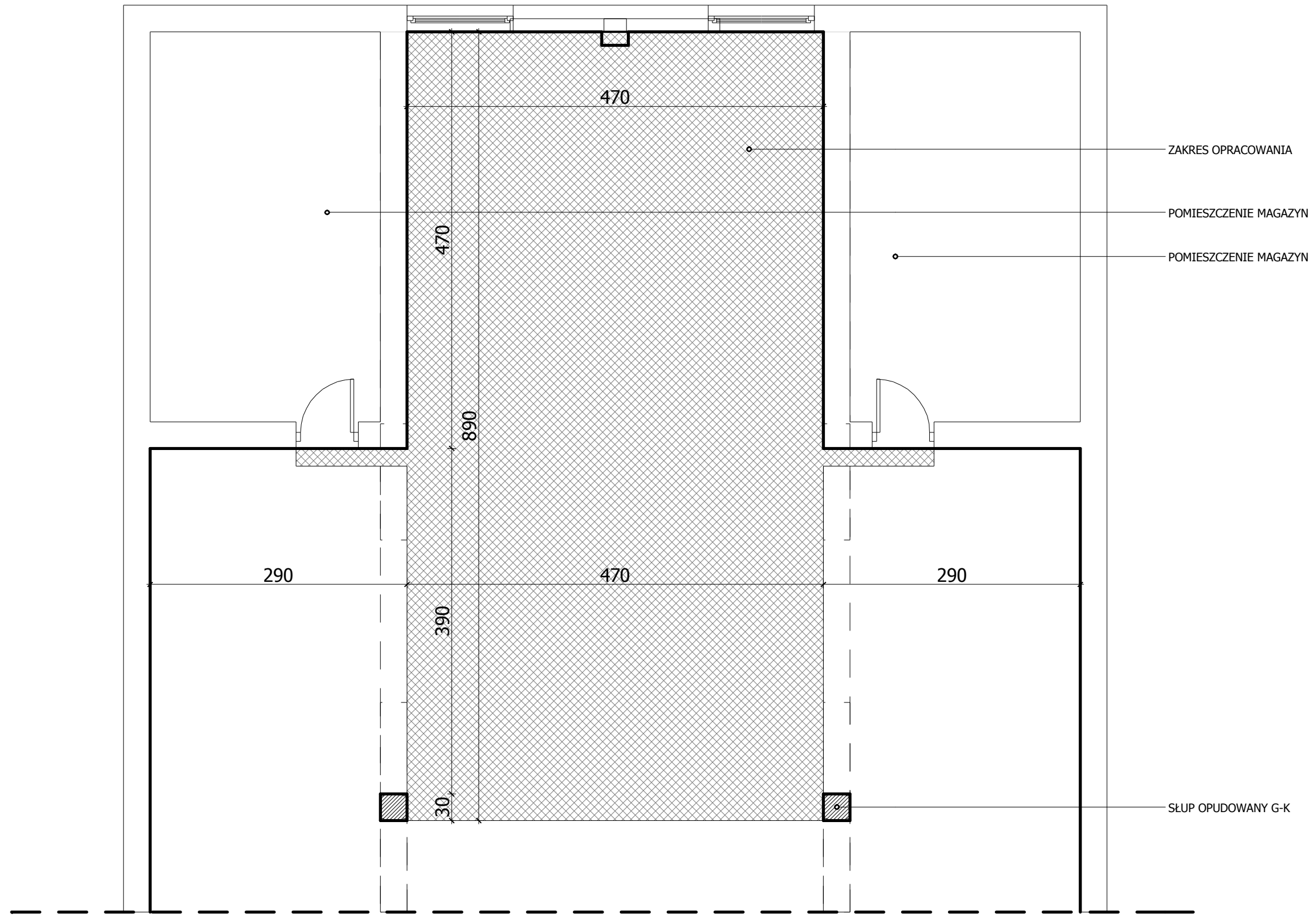
KONDYGNACJA+2 (PODDASZE)
