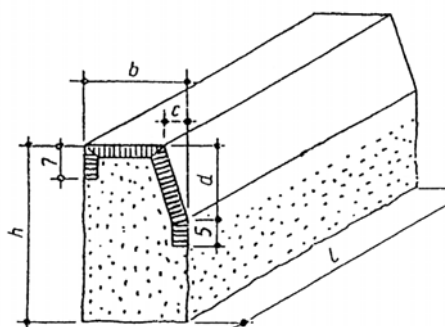
Krawężnik uliczny rodzaju A
