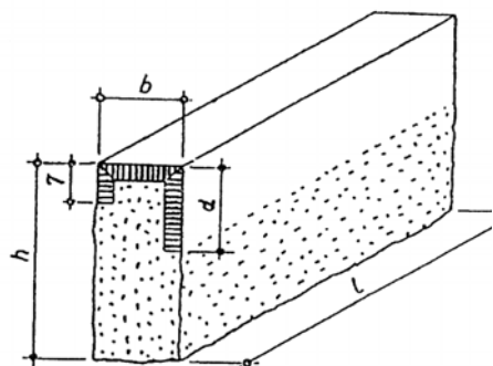
Krawężnik uliczny rodzaju B
