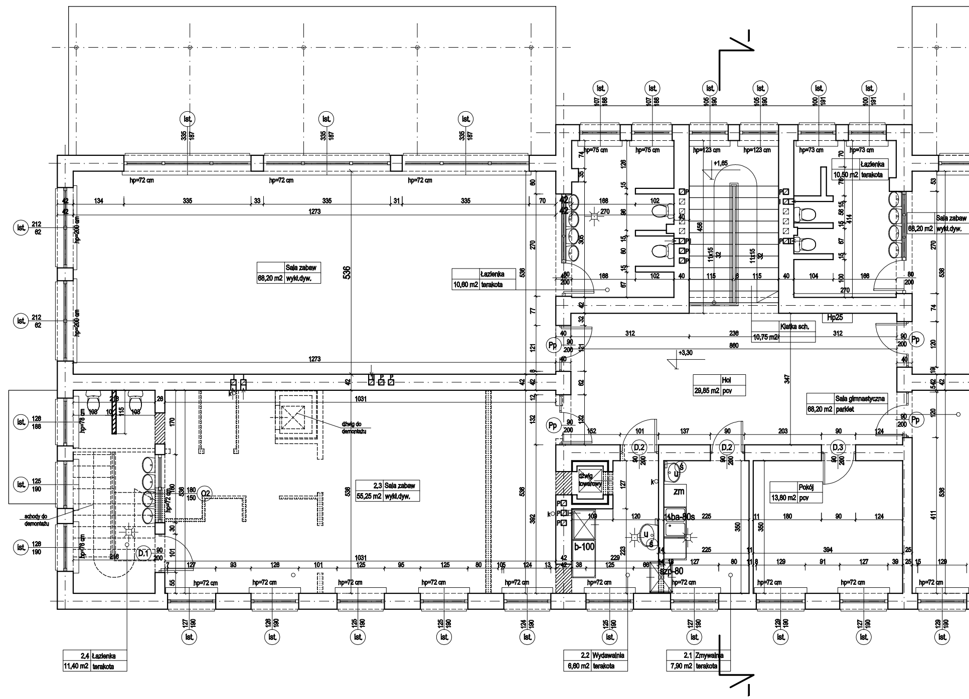
TECHNOLOGIA RZUT PIĘTRA ( fragment ) 1:100
