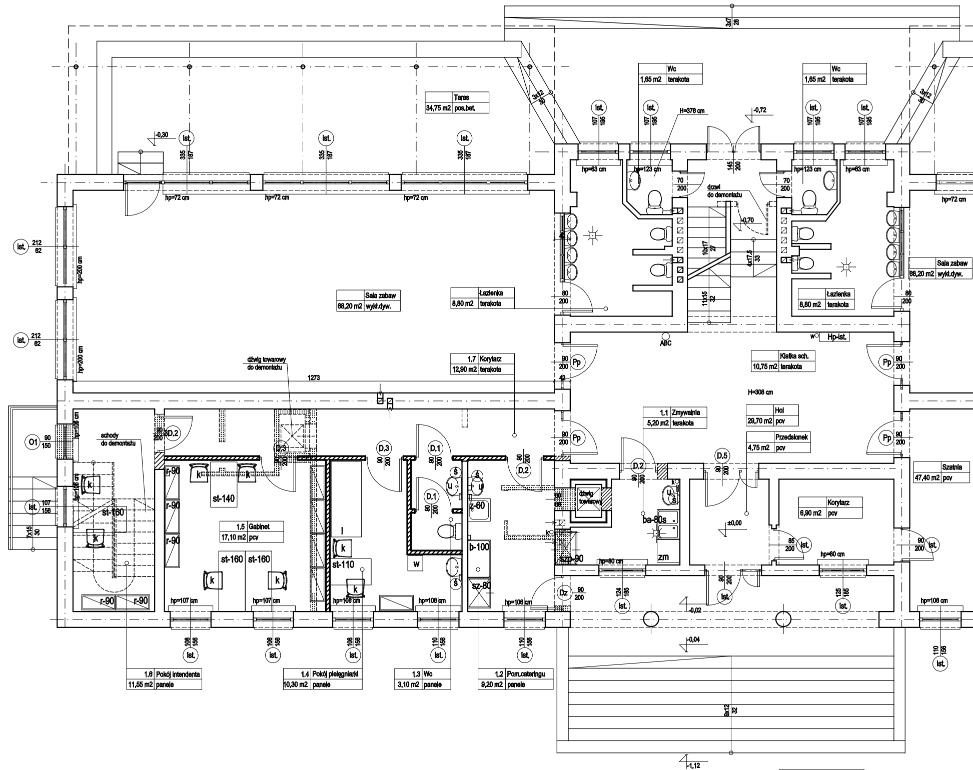
TECHNOLOGIA RZUT PARTERU ( fragment ) 1:100
