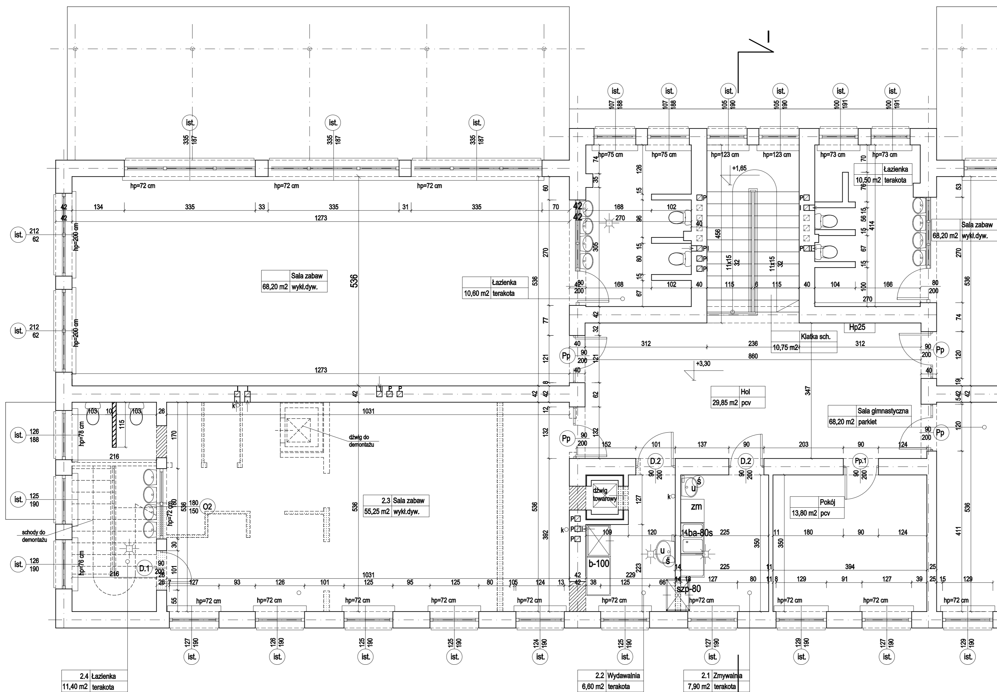
RZUT PIĘTRA 1:50
