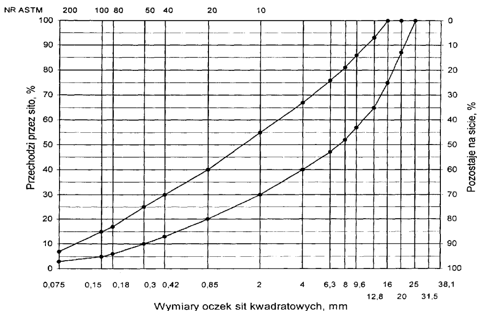
Rys. . Krzywe graniczne uziarnienia mieszanki mineralnej BA od 0 do 20 mm do warstwy wiążącej, wyrównawczej i wzmacniającej nawierzchni drogi o obciążeniu ruchem KR1 lub KR2
