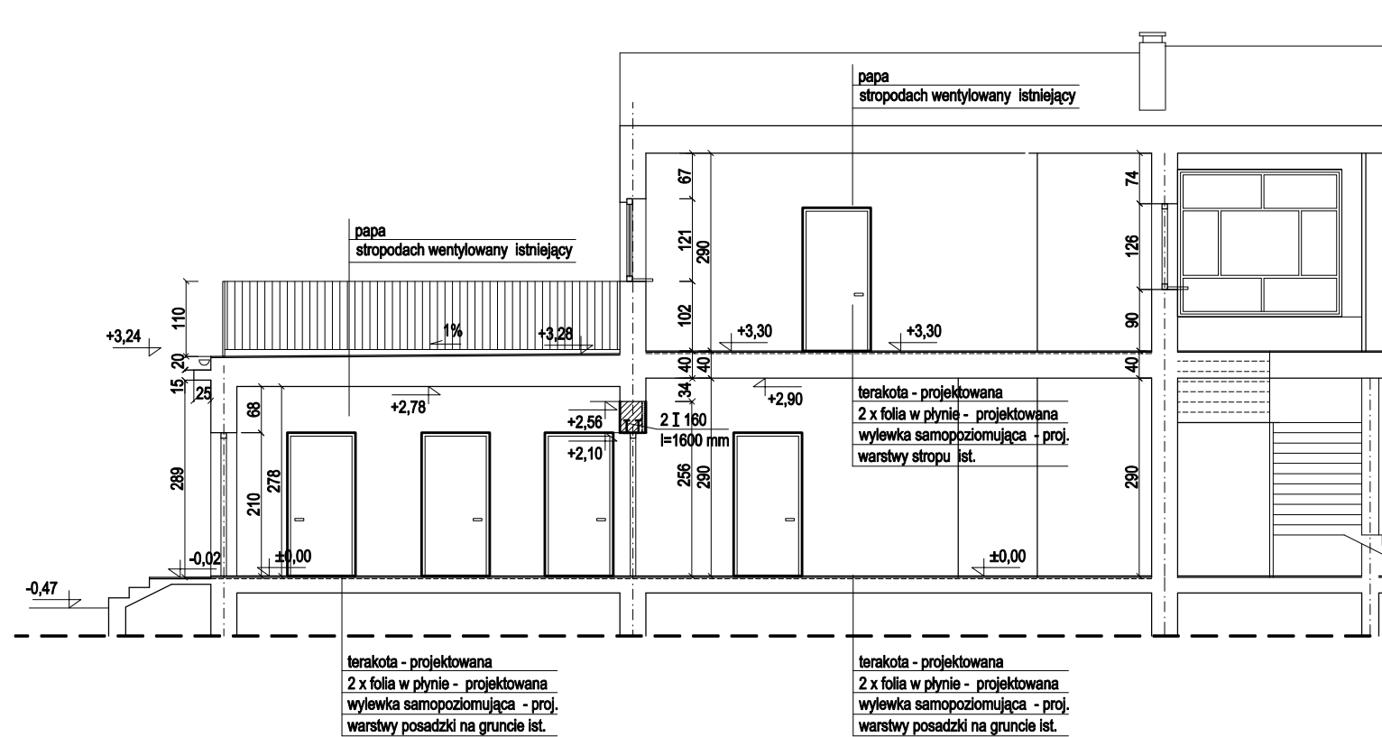
PRZEKRÓJ I-I 1:100
