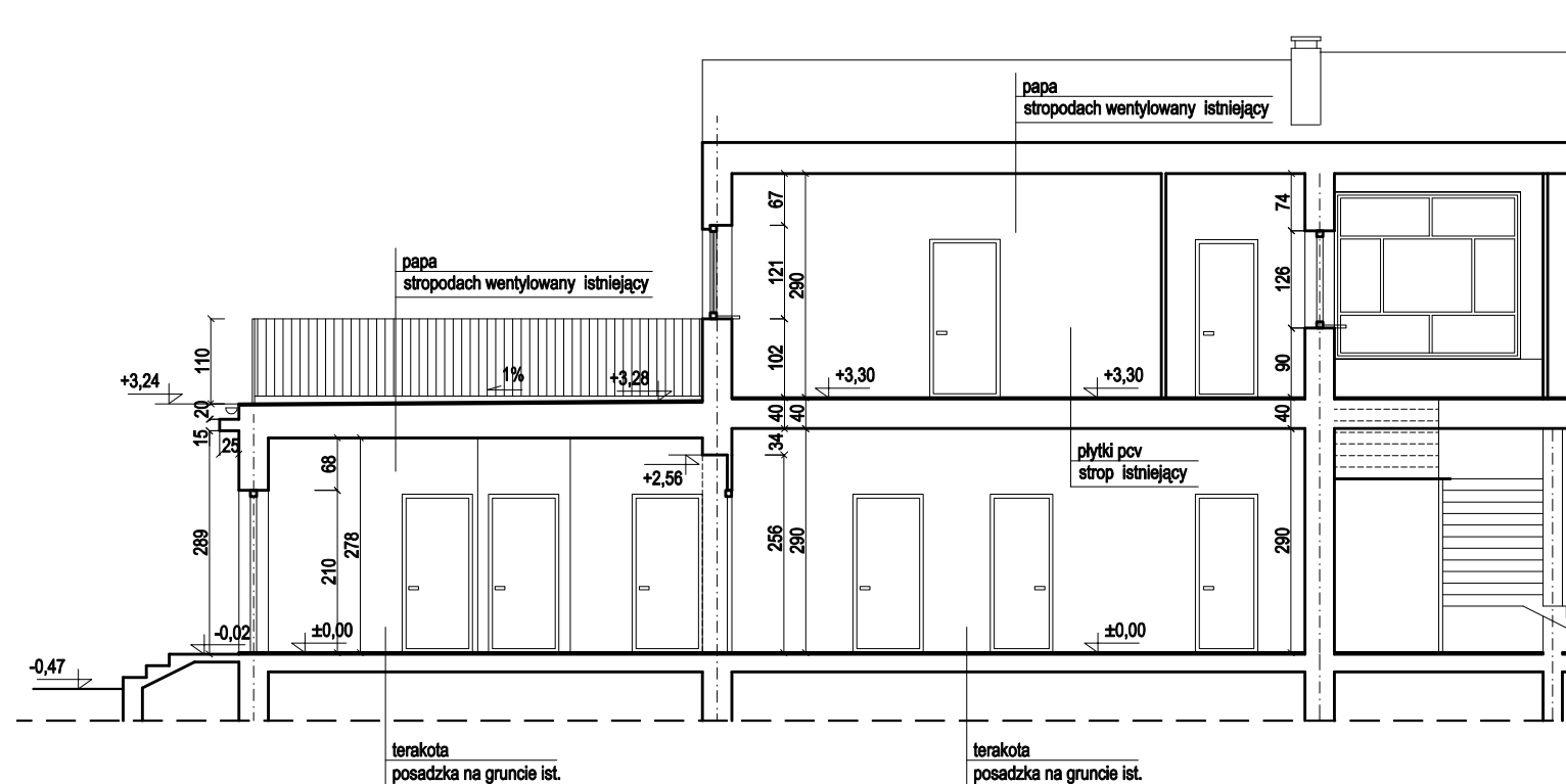
PRZEKRÓJ I - I 1:100
