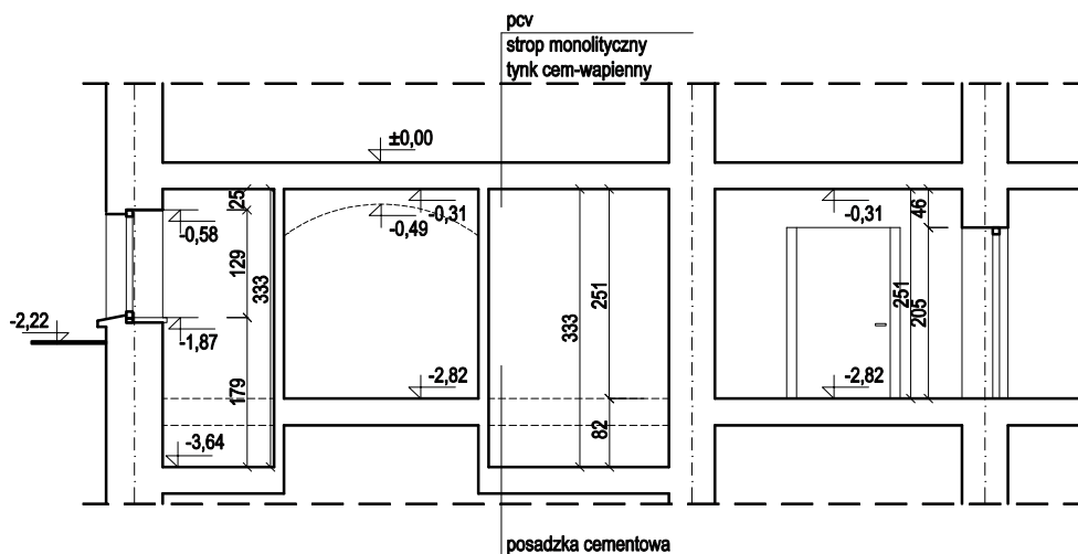
PRZEKRÓJ II - II 1:100
