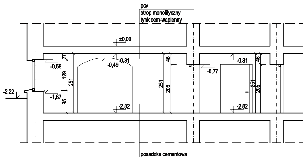
PRZEKRÓJ I - I 1:100
